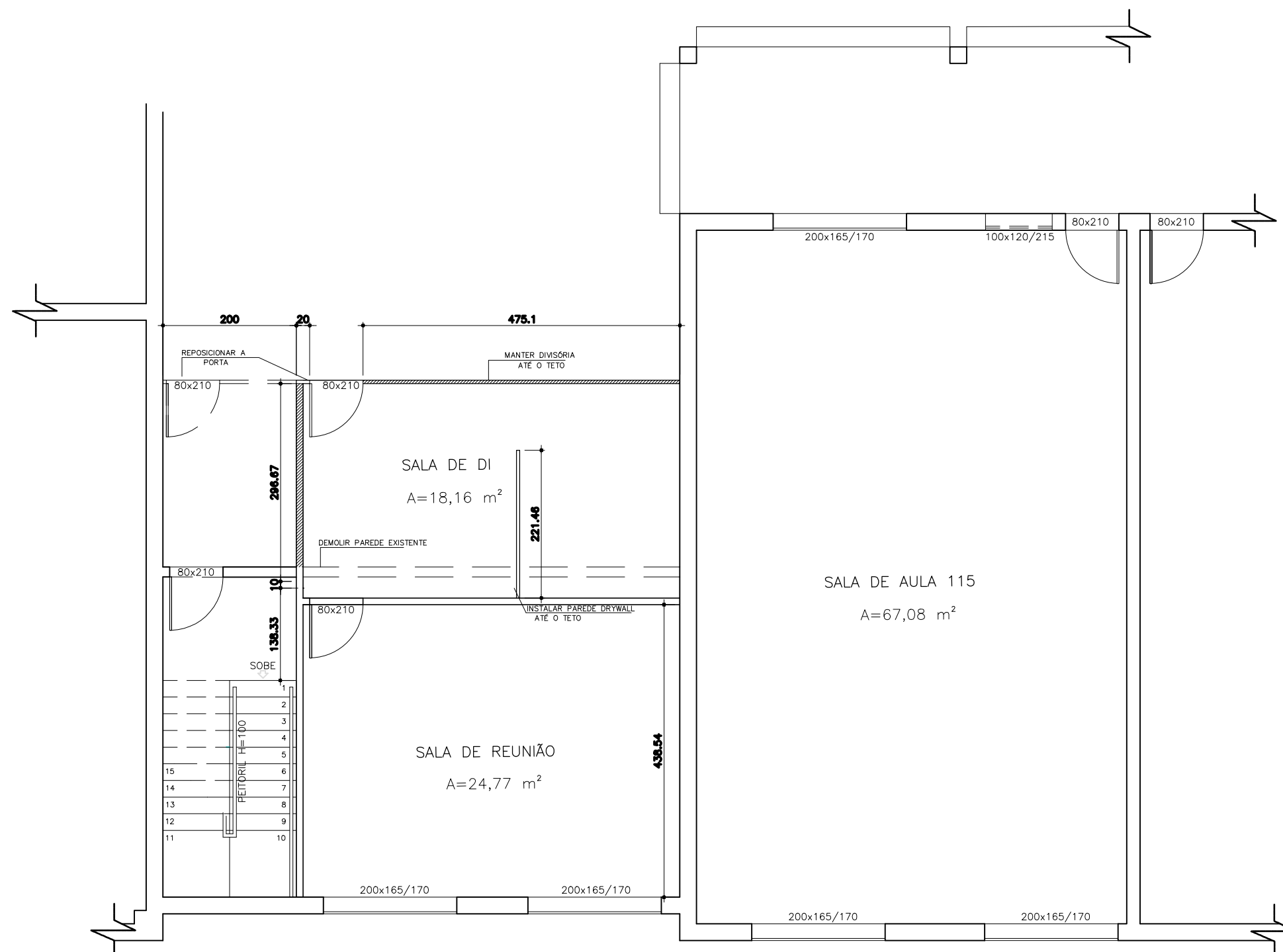
PLANTA EXECUTIVA (COTAS) ESCALA 1:75
