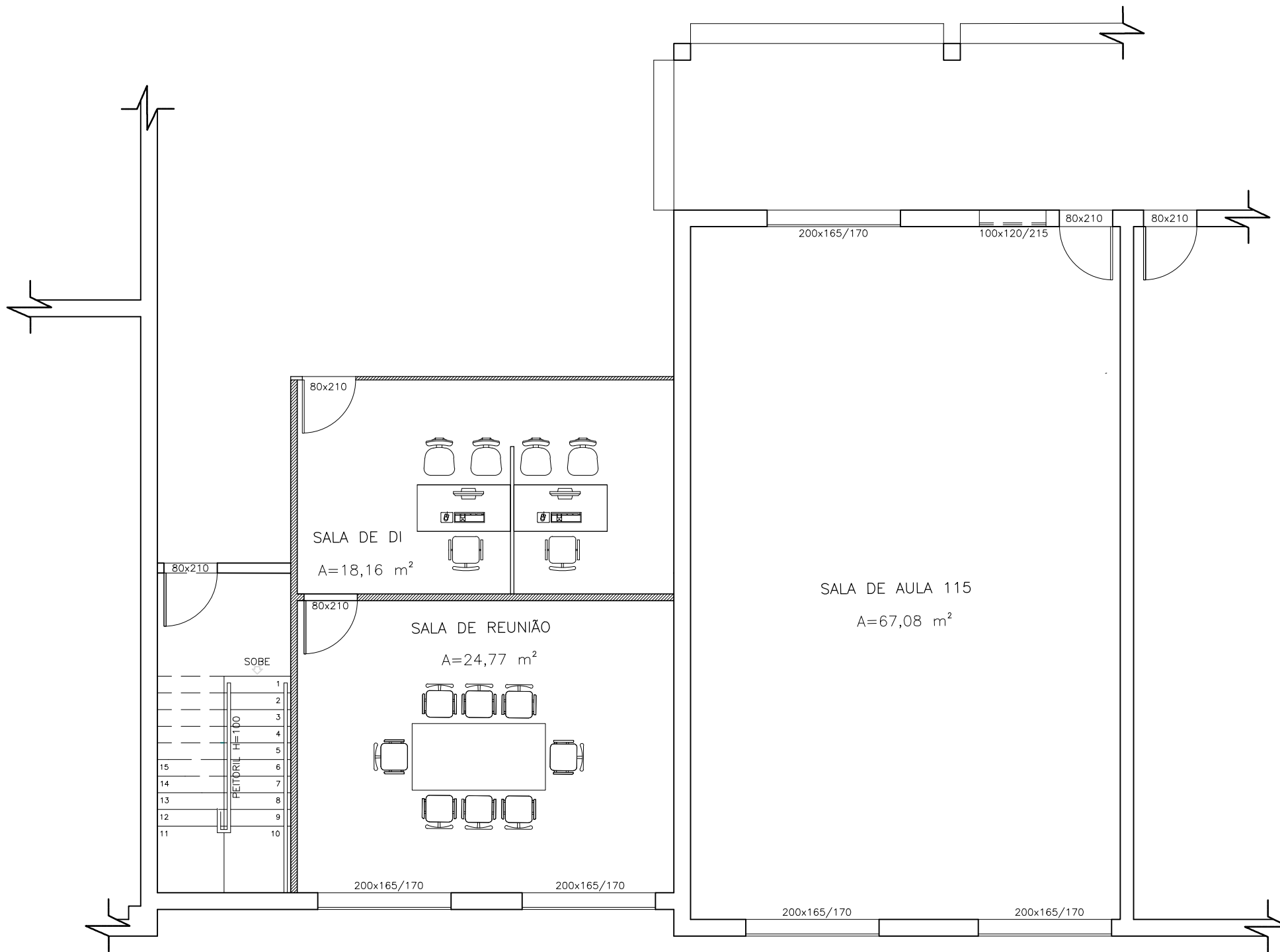
PLANTA LAYOUT ESCALA 1:75
